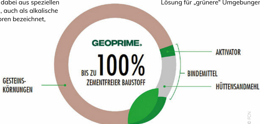
Zusammensetzung der FCN-Klimabetonpflastersteine.
