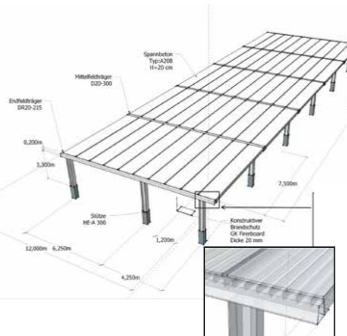
1c: Variante A315 BRESPA®-Decke A20B, 20 cm Flachdecke, Spannrichtung längs (Spannweiten: 7,50 m)
