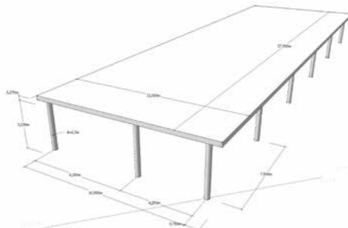
1a: Variante A310 - Stahlbetondecke, 27 cm Flachdecke, (Spannweiten: 6,25 m / 4,25 m)
