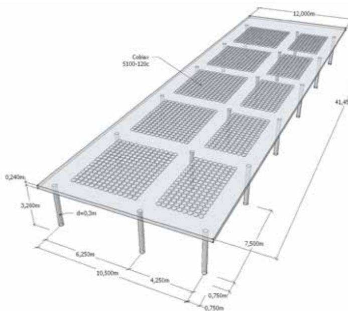
1b: Variante A319 - Cobiax-Decke, 24 cm Flachdecke (Spannweiten: 6,25 m / 4,25 m)
