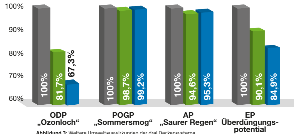
Abbildung 3: Weitere Umweltauswirkungen der drei Deckensysteme im Vergleich (Quelle: S. Wünschmann)
