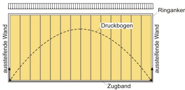
Bogen-Zugbandmodell:
