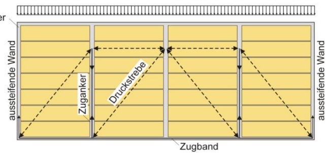
Fachwerkmodell:
